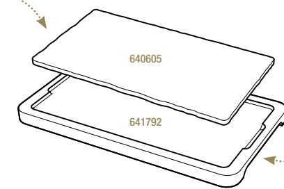
PLATEAU POUR ASSIETTE 30 x 16 CM LINER TRAY FOR PLATE 11 3/4 x 6 1/4"
